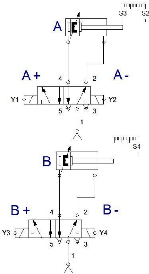
Diagrama de Potencia
