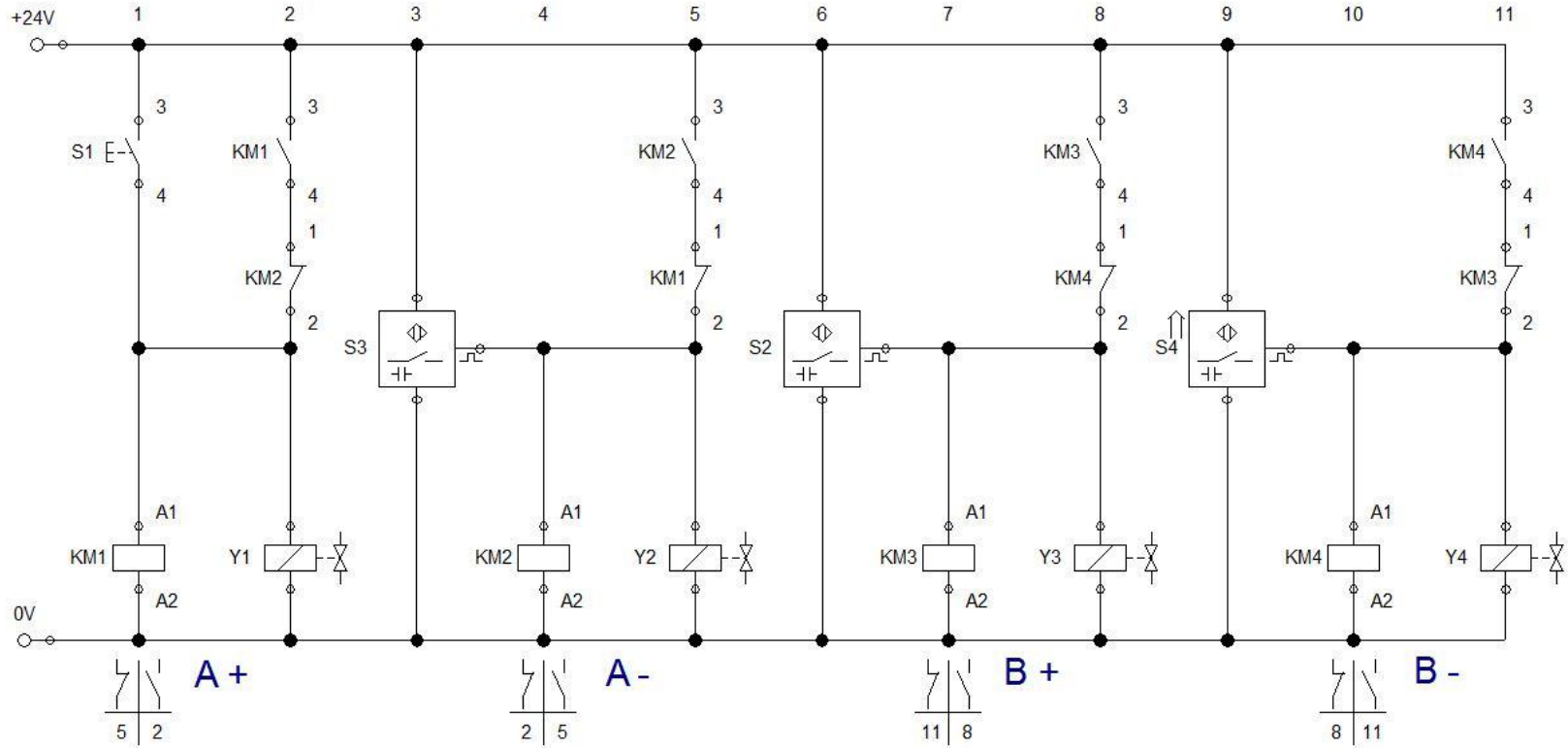
Diagrama de Mando y Control
