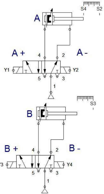
Diagrama de Potencia
