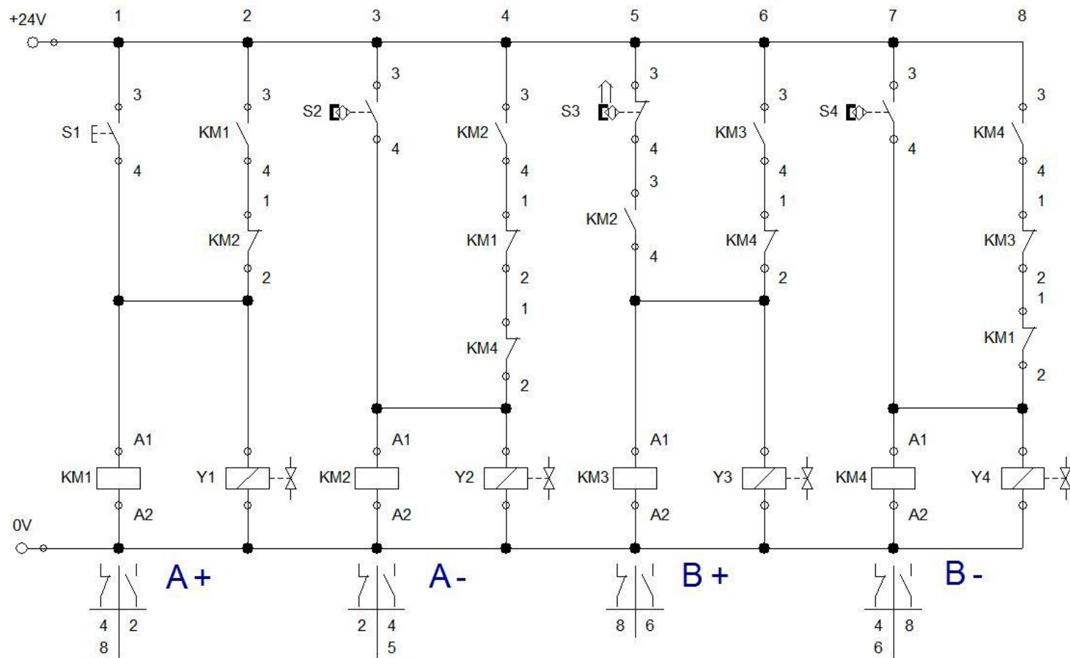
Diagrama de Mando y Control
