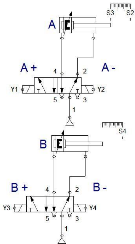
Diagrama de Potencia
